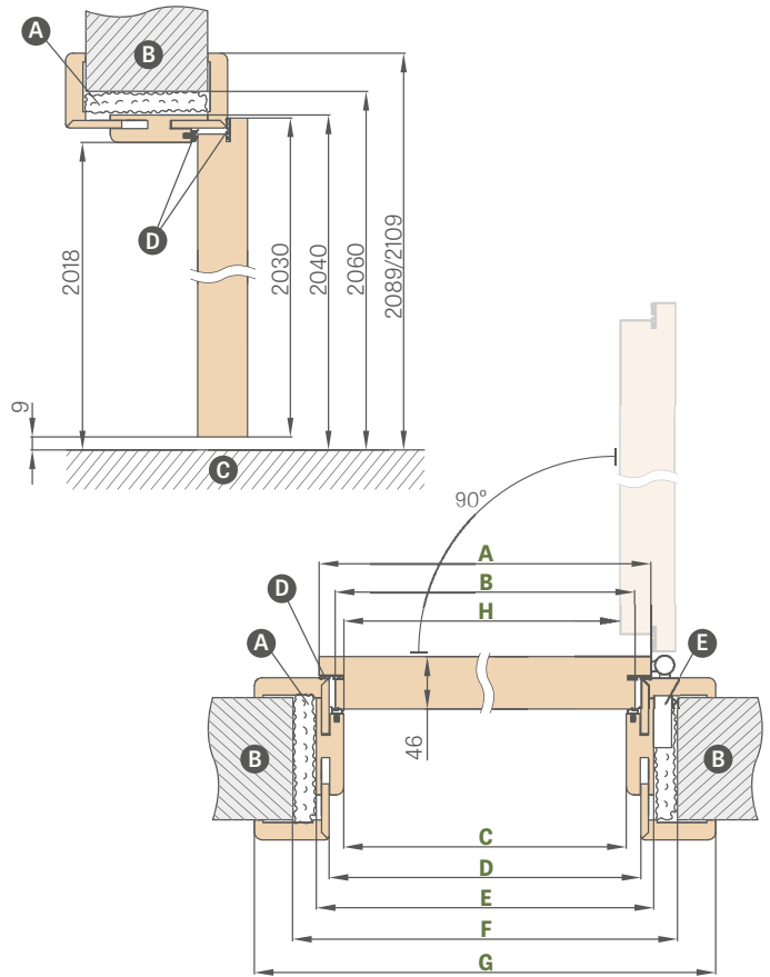
HERSE SET ÁLLÍTHATÓ AJTÓTOK KERESZTMETSZETE
